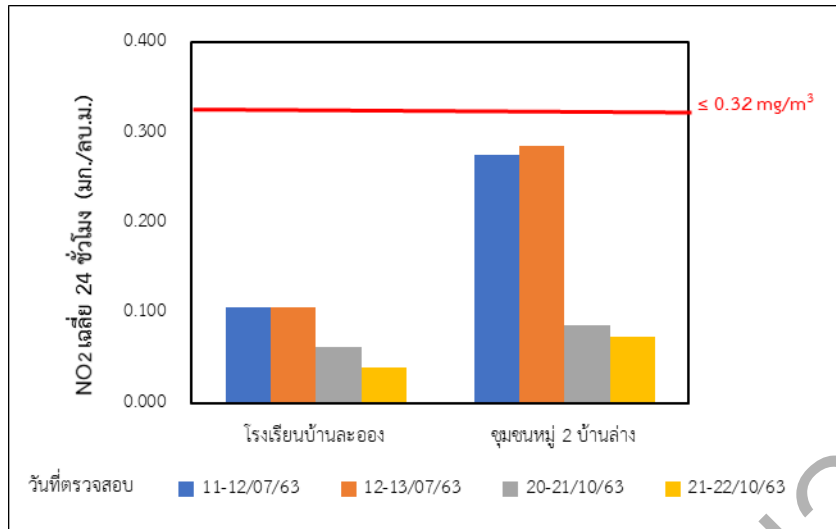
รูปแสดงผลการตรวจวัดคุณภาพอากาศบริเวณพื้นที่ศึกษาท่าอากาศยานระนอง (NO 2 )
